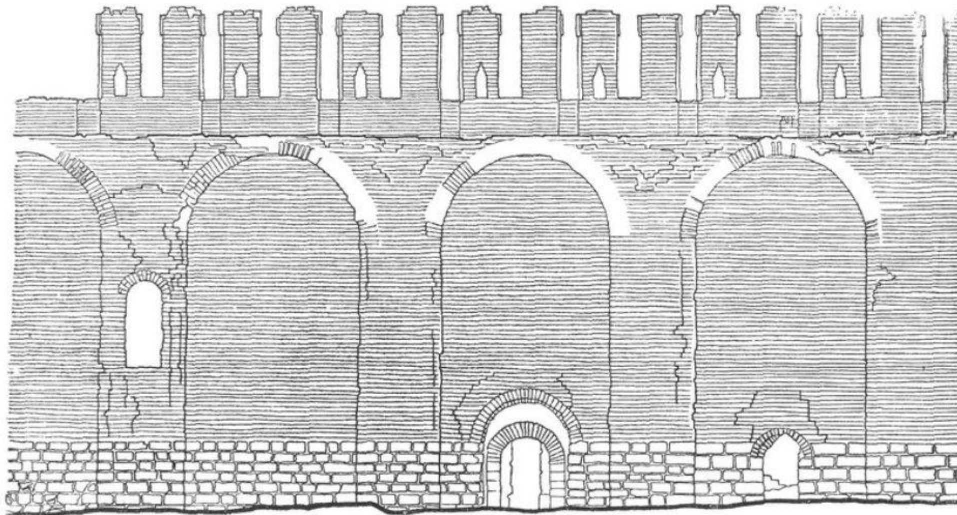
Арки тыльной стороны стены Смоленской крепости (Обмер РСНРПМ)
